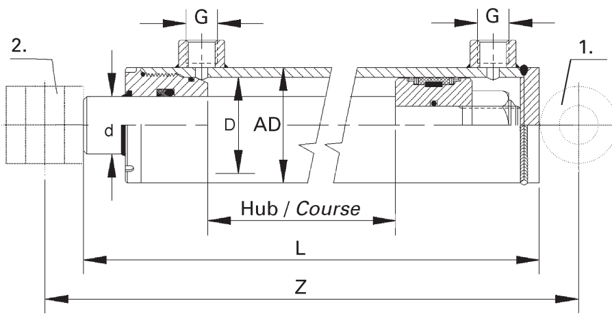
Doppelwirkender Zylinder
