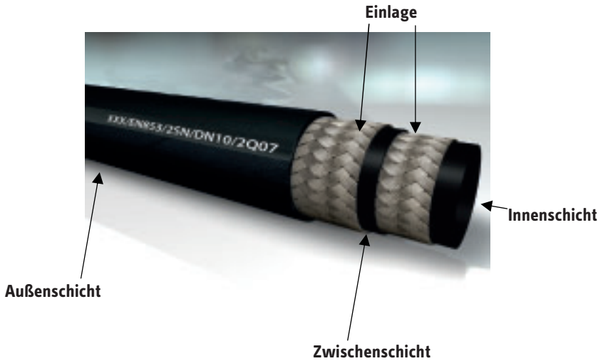
Abbildung 1: Hydraulikschlauch
