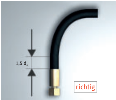
Abbildung 8: richtig - Gerader Abschnitt mit 1,5 d_a vor Biegung falsch - Eine Schlauchscheuerschutzspirale stellt keinen Knickschutz dar
